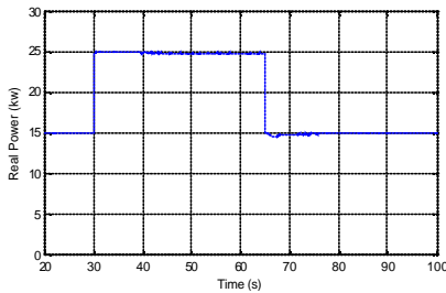
Fig. 8.b: P_{bhta}
