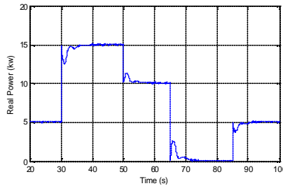
Fig. 9.b: P_{bhta}
